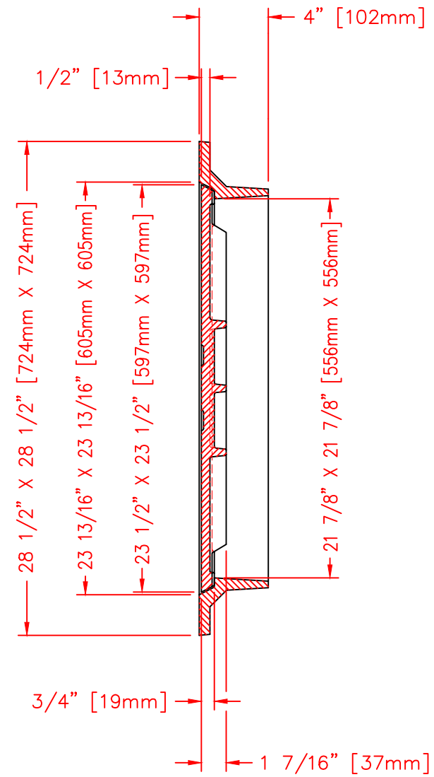
SECTION A-A
