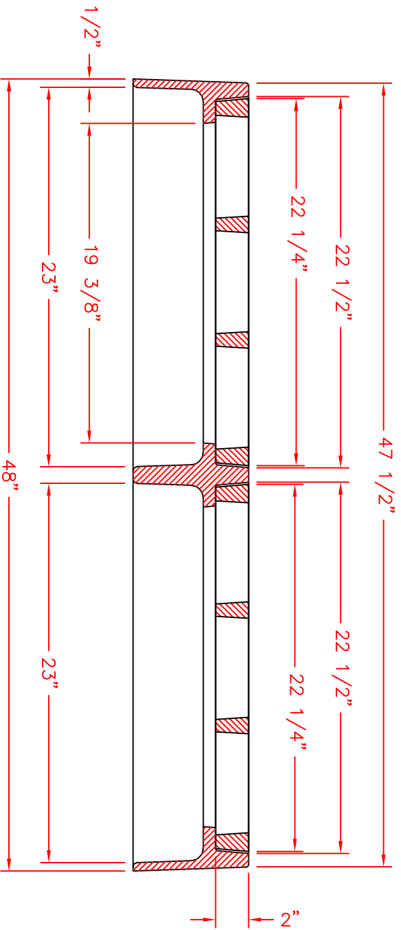
SECTION A-A
